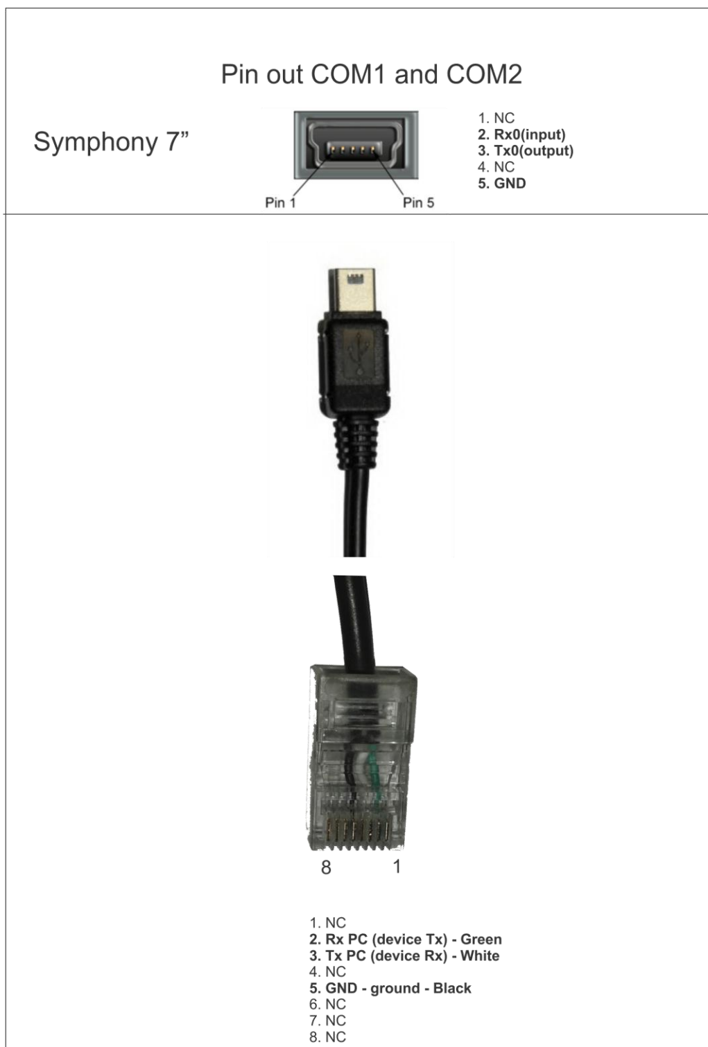
Slika 4 – Opis serijskog kabla za povezivanje uređaja Symphony 7" sa HCP fiskalnim uređajima (mini USB na RJ45)
