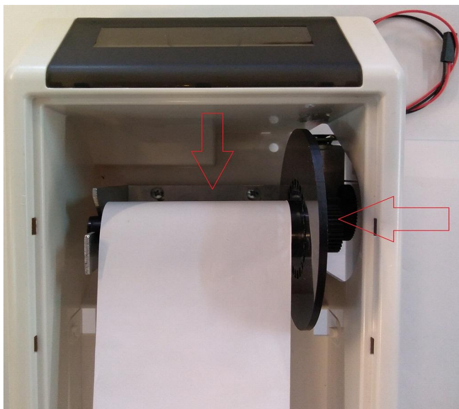
Slika 6: Postavljanje plasti nog kalema i termalnog papira
