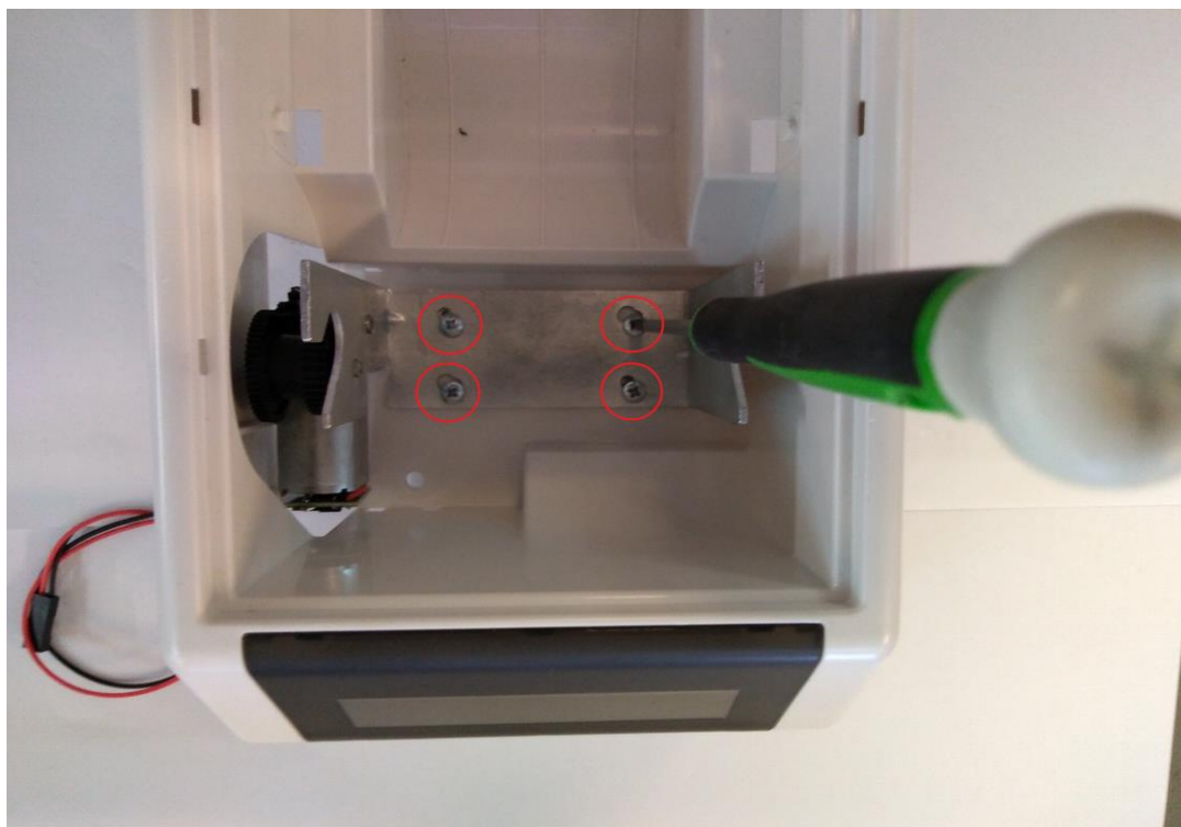
Slika 4: Pričvršćivanje sklopa namotača
