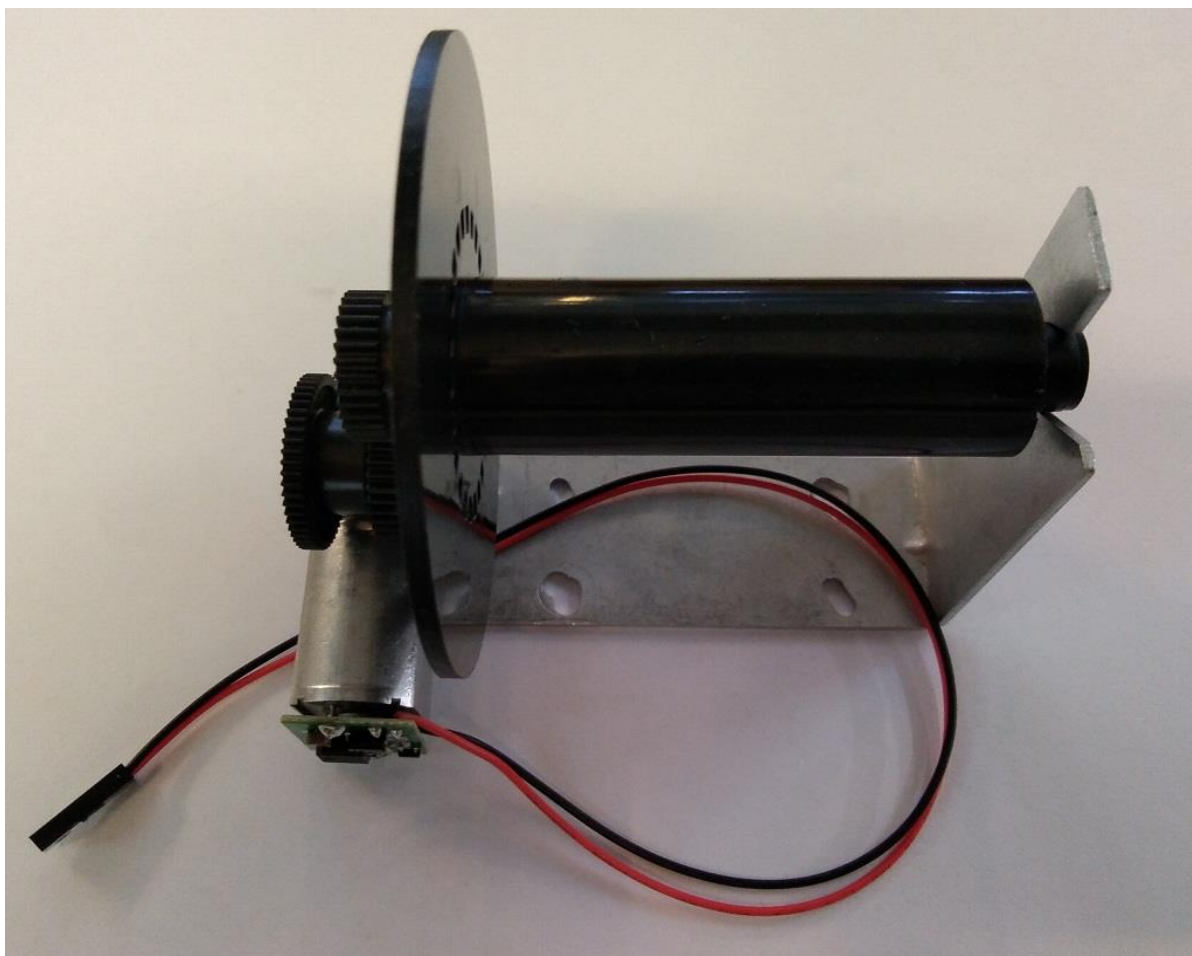
Slika 2: Izgled sklopa namotača
