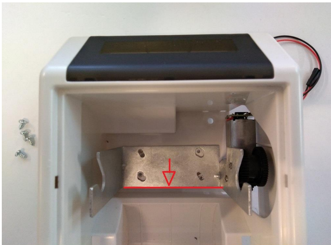
Slika 3: Postavljanje sklopa namotača
